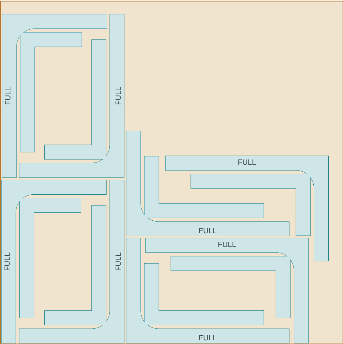
LAYER 1 - L1 course 7
