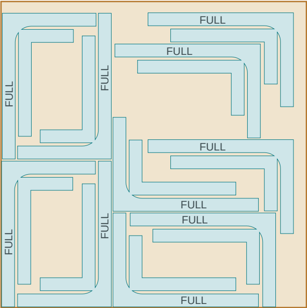
LAYER 4 - L1 course 1
